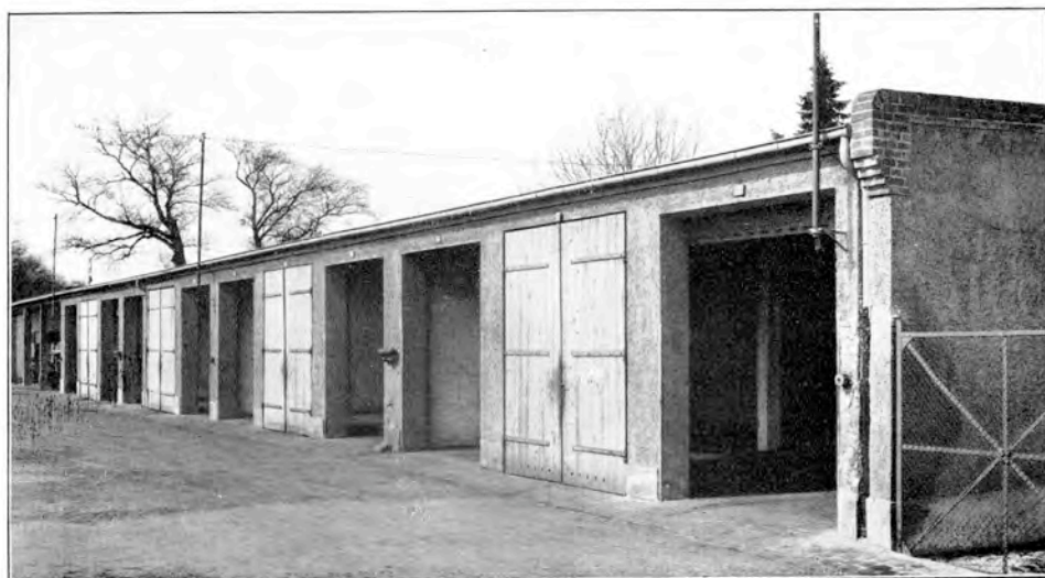
Olex-Garagen, Rummelsburg, Tankanlage Nobelshof. Architekt: Techn. Büro „Olex“.
